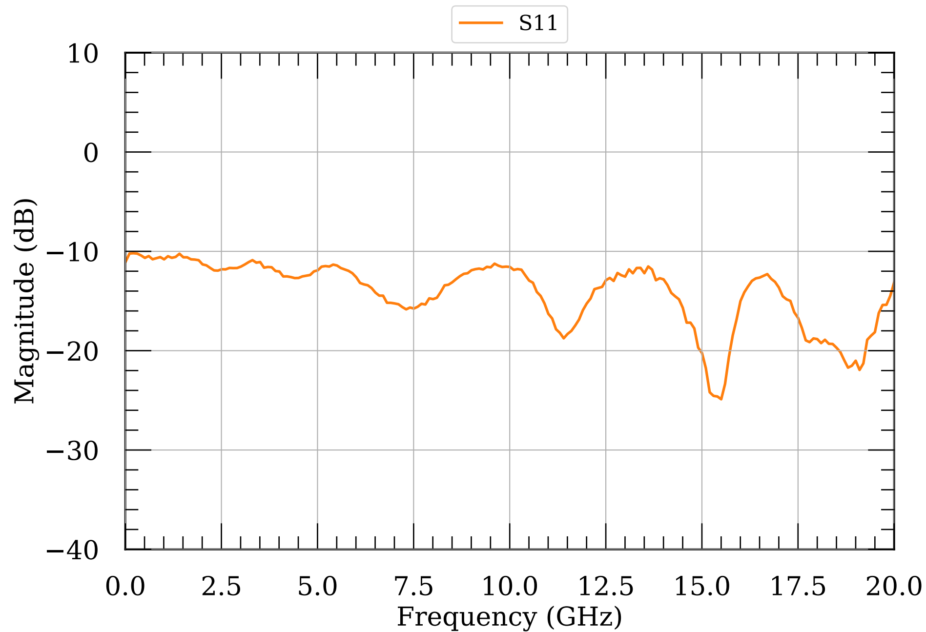
LNA S-params module061
